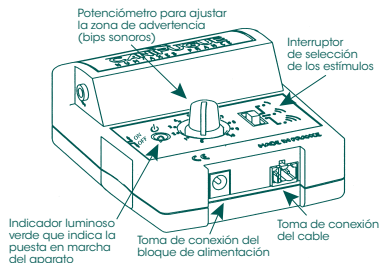
Esquema n° 1: caja emisora
