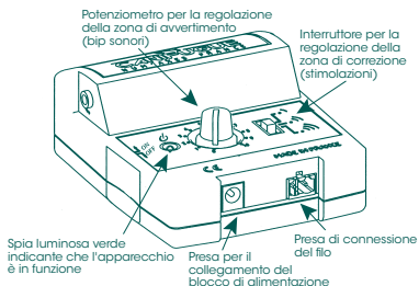
Schema n° 1 : centralina emittente
