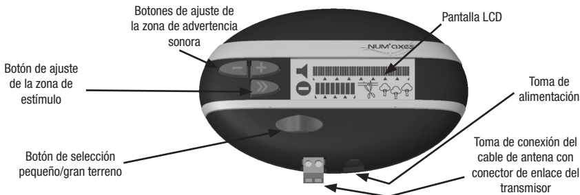
Fig. 1 – Transmisor
