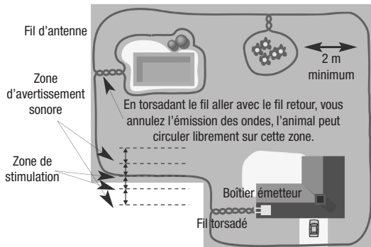
Fig. 4 – Exemple d'installation
