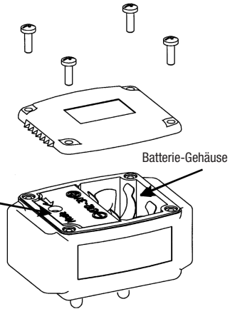
Abb. 3 – Empfänger-Halsband
