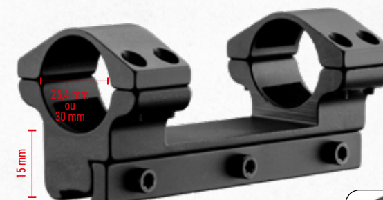
Montage monobloc Gamo
