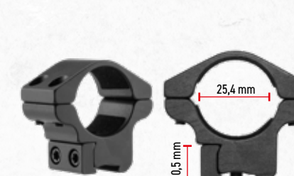
Montage bas ø 25,4 mm sur rail prisme 11 mm
