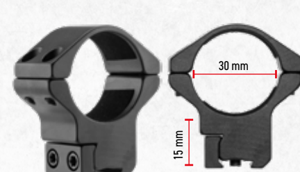
Montage Moyen ø 30 mm sur rail prisme 11 mm
