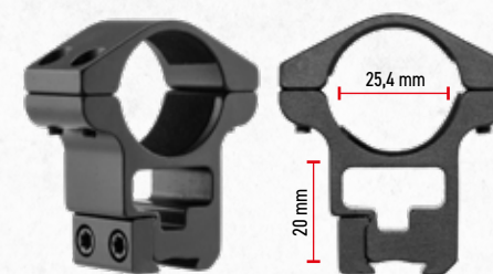
Montage haut avec tunnel de visée ø 25,4 mm sur rail prisme 11 mm
