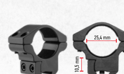
Montage Moyen ø 30 mm sur rail prisme 11 mm
