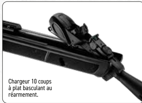
Bascule du canon : réarme le piston IGT et positionne le plomb suivant pour le tir.
