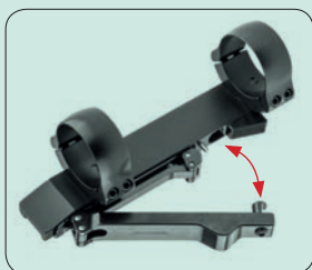
Colliers standards , spéciaux, à démontage rapide...
